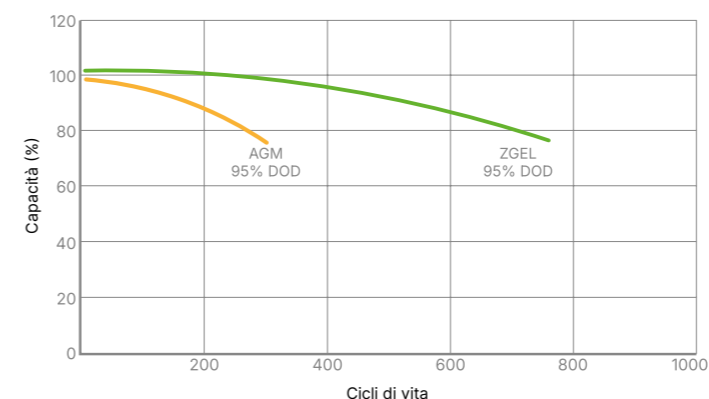
Zenith ZGEL vs Standard AGM Test cicli di vita con 95% D.O.D.
